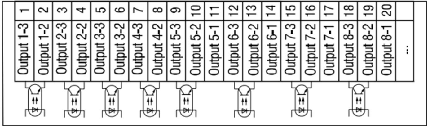
IESIRI PE TRANZISTOR NPN ; TRM138-T
