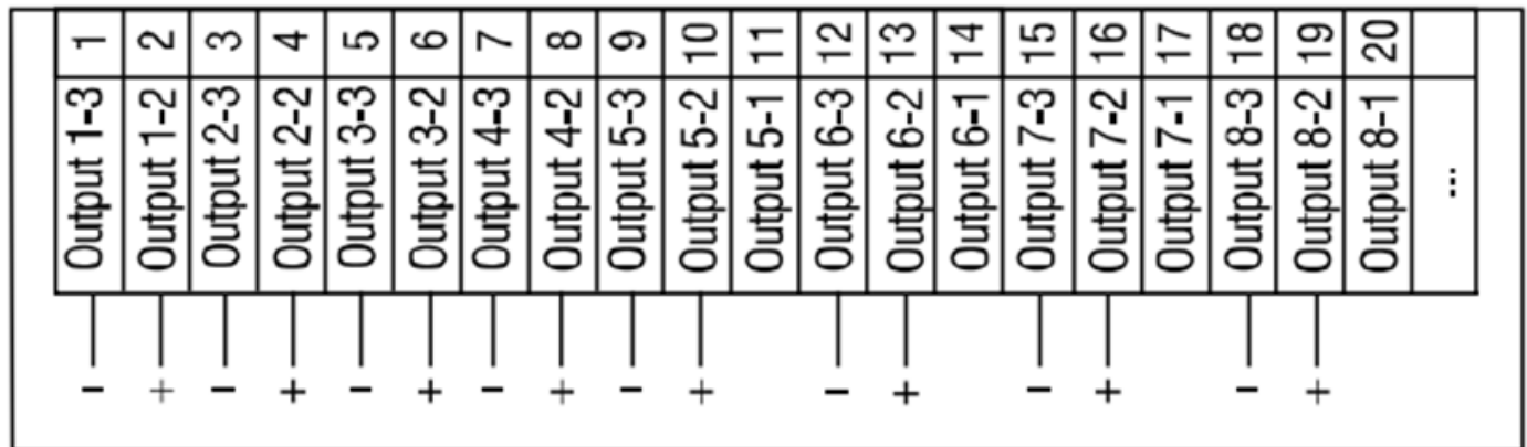
IESIRI de COMANDA pentru RELEE SOLID STATE - SSR ; TRM138-S si IESIRI ANALOGICE de RETRANSMISIE 4-20 mA ; TRM138-I
